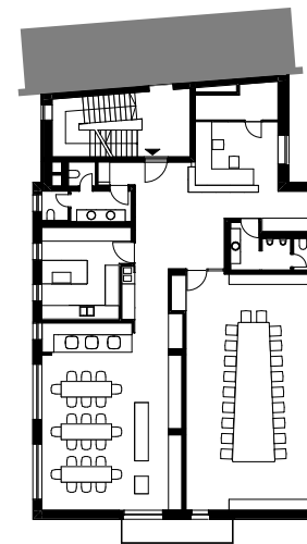
Grundriss
